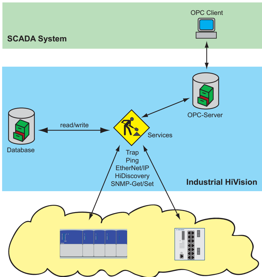
Abb. 50: Anbindung an Prozessvisualisierungssystem
