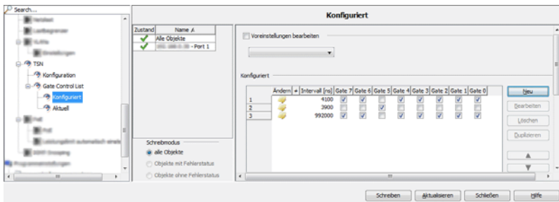
Abb. 44: Gerät 1 TSN > Gate Control List > Konfiguriert
