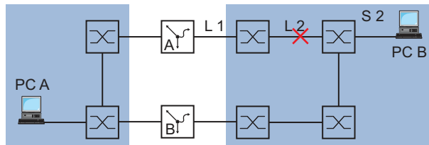
Abb. 67: Überwachen einer Leitung mit Ping-Tracking
