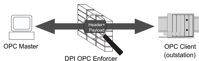
Abb. 25: Inspektion der Datenpakete
