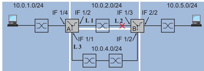
Abb. 70: Statisches Route-Tracking konfigurieren
