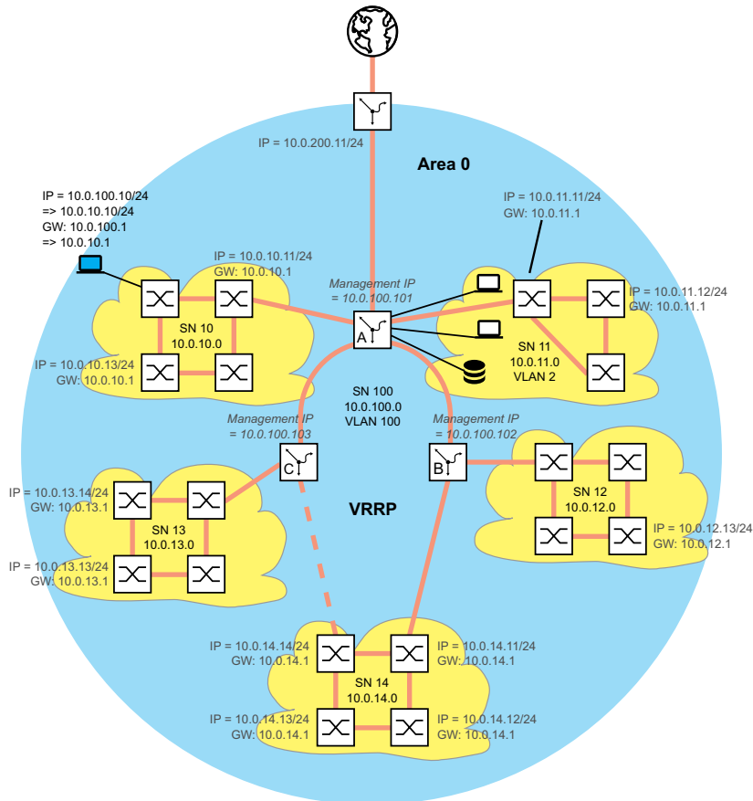
Abb. 64: Netzplan mit Management-IP-Adressen
