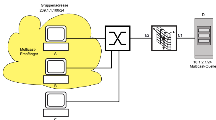
Abb. 62: Beispiel für statisches Multicast-Routing
