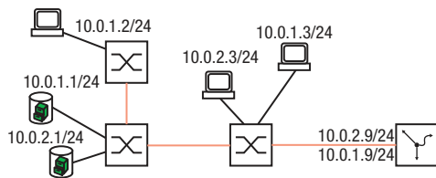
Abb. 40: Beispiel für Multinetting
