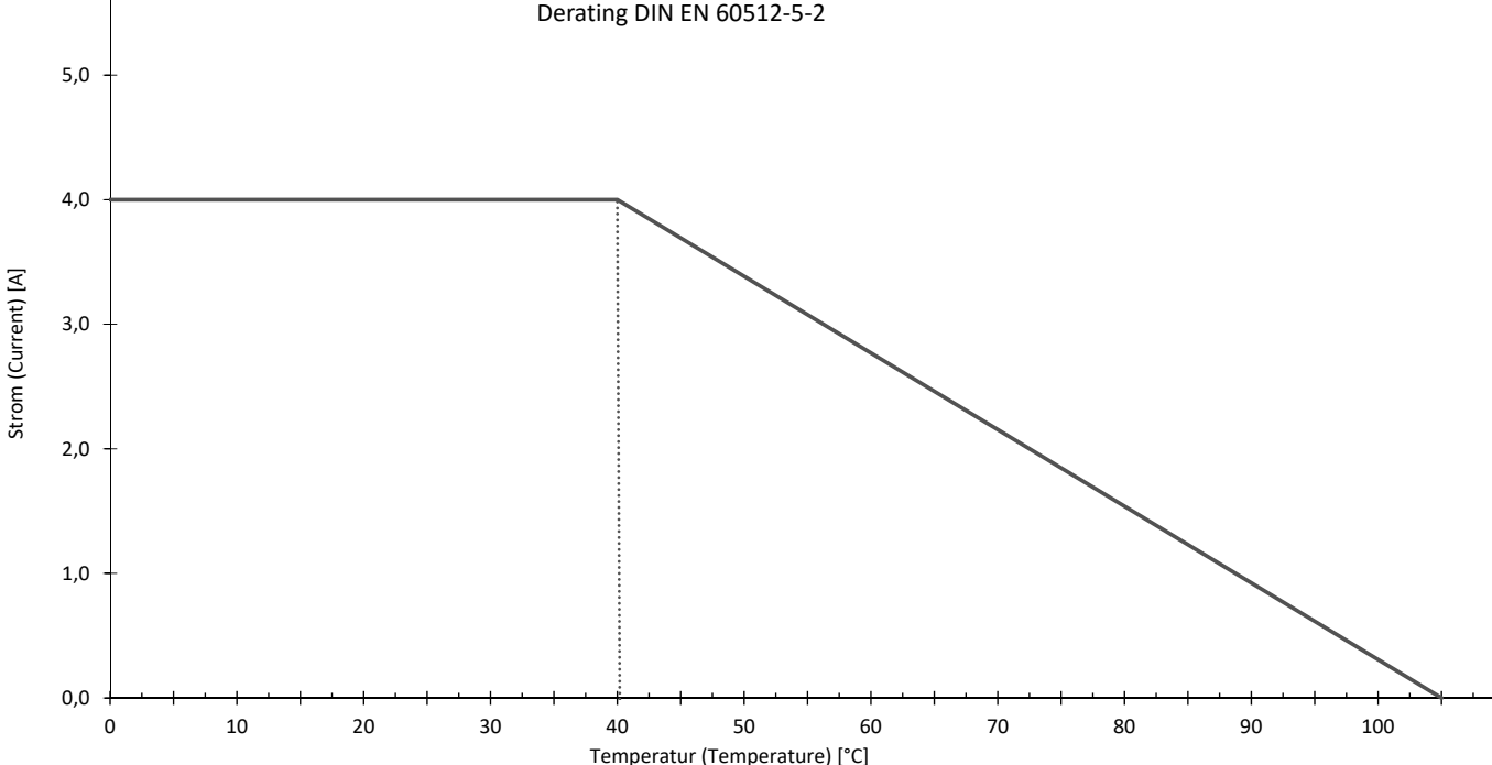
Derating DIN EN 60512-5-2
