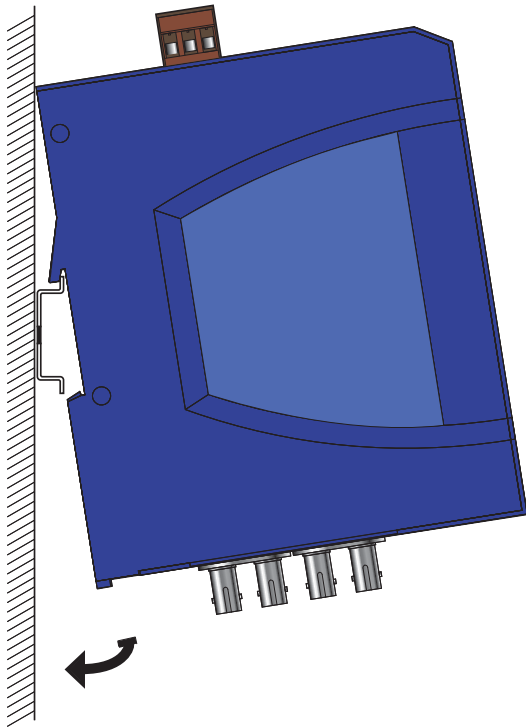
Abb. 3: Montage auf die Hutschiene
