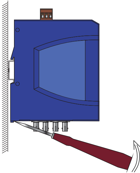
Abb. 4: Demontage von der Hutschiene
