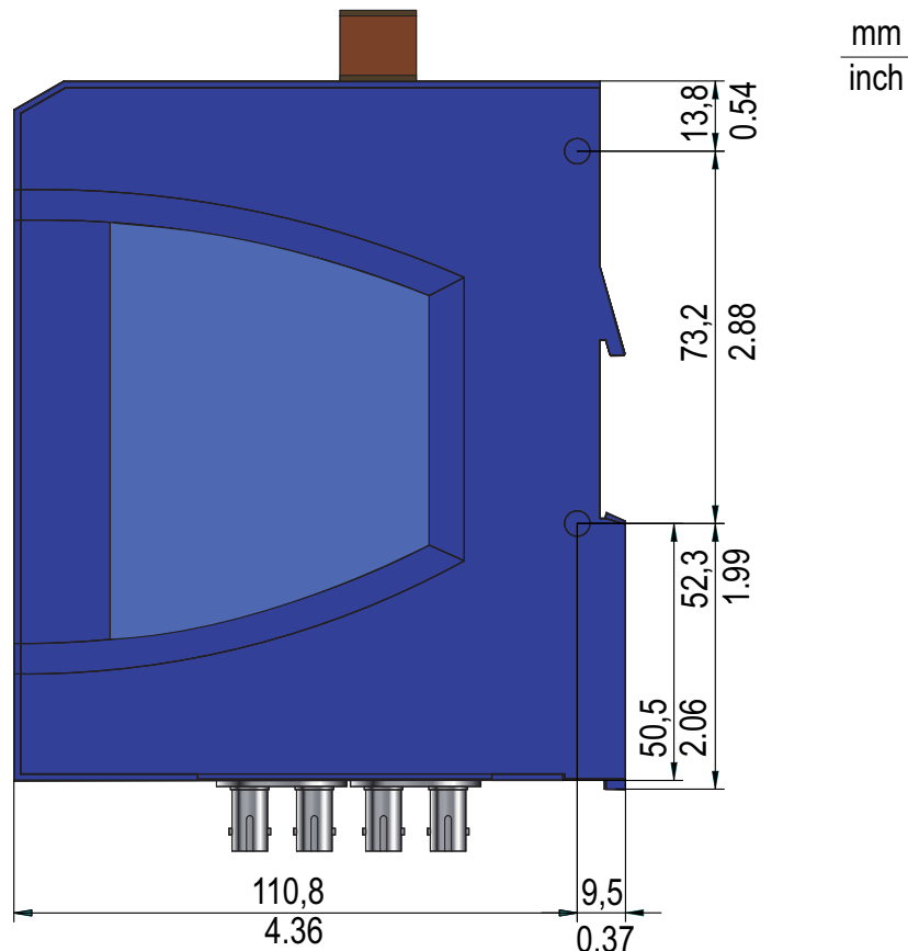
Abb. 7: Abmessungen des SPIDER II
