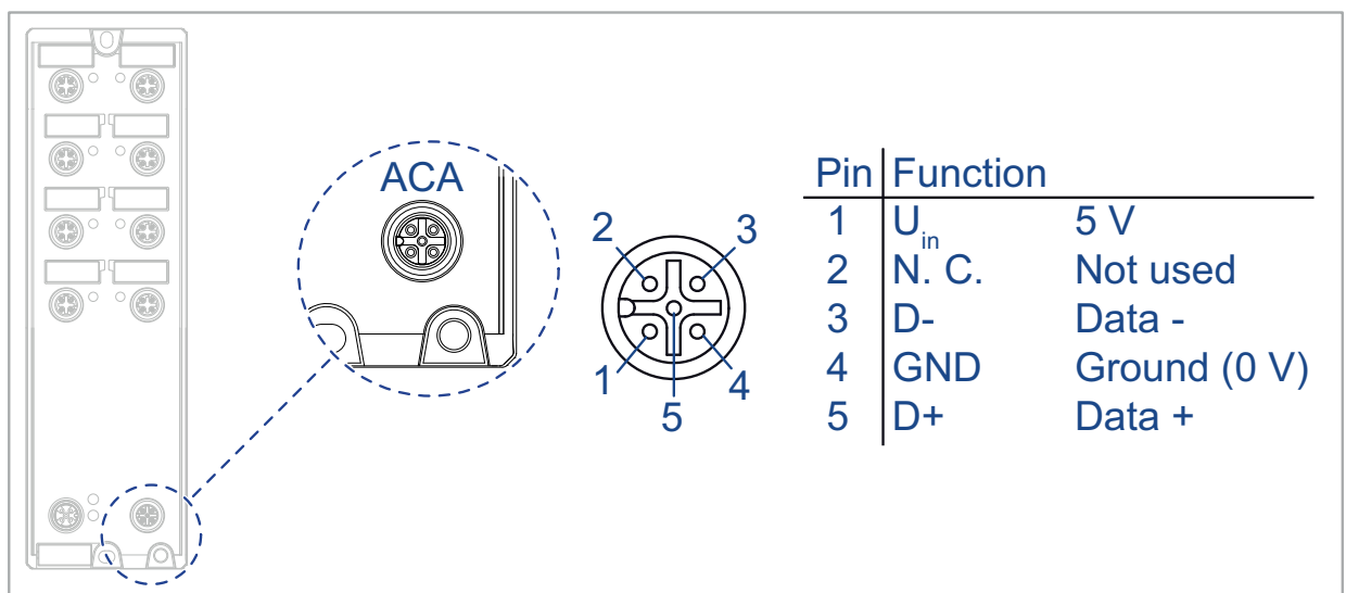
Abb. 7: ACA-M12-Schnittstelle
