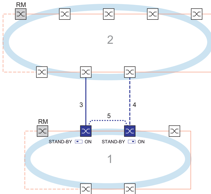
Abb. 57: Beispiel für die 2-Switch-Kopplung mit Steuerleitung
