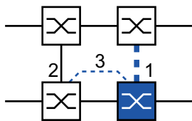
Abb. 51: 2-Switch-Kopplung mit Steuerleitung, Standby-Gerät
