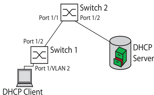
Abb. 61: Beispiel: DHCP-Schicht-2-Netz
