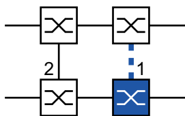
Abb. 56: 2-Switch-Kopplung, Standby-Gerät 1: Kopplungs-Port 2: Partner-Kopplungs-Port
