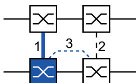
Abb. 58: 2-Switch-Kopplung mit Steuerleitung, primäres Gerät 1: Kopplungs-Port 2: Partner-Kopplungs-Port 3: Steuerleitung
