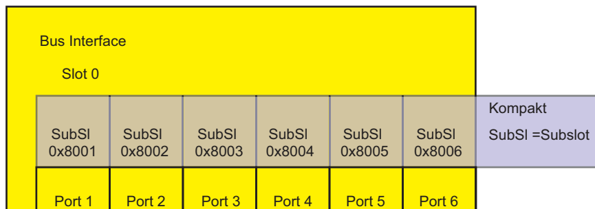
Abb. 70: Kompaktes Gerät
