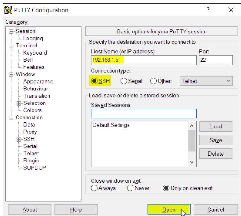
Abb. 89: PuTTY-Eingabemaske
