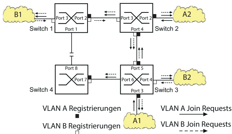
Abb. 63: MVRP -Beispiel-Netz für VLAN-Registrierung
