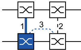
Abb. 50: 2-Switch-Kopplung mit Steuerleitung, primäres Gerät
