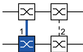
Abb. 55: 2-Switch-Kopplung, primäres Gerät 1: Kopplungs-Port 2: Partner-Kopplungs-Port
