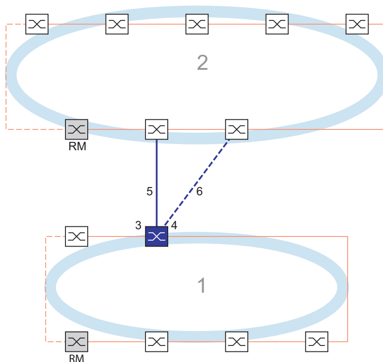
Abb. 52: Beispiel für die 1-Switch-Kopplung
