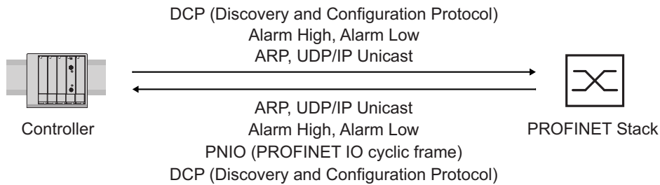
Abb. 69: Kommunikation zwischen Controller und dem Gerät
