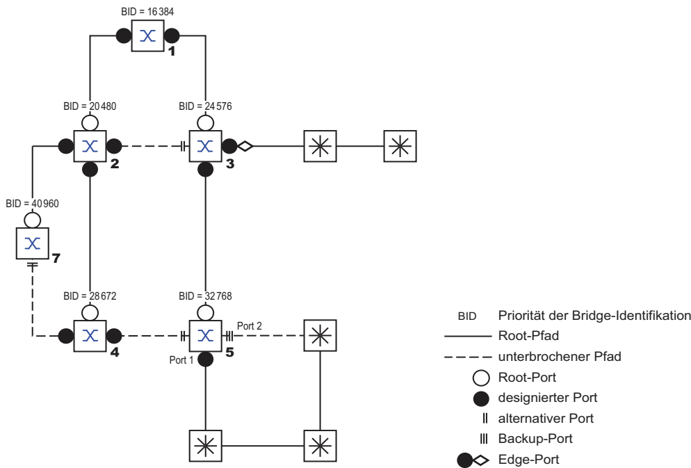
Abb. 49: Port-Rollen-Zuweisung
