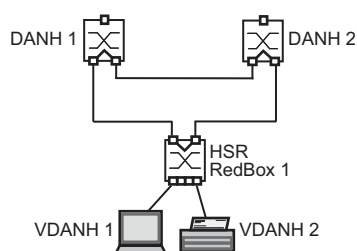
Abb. 38: VDANH mit einem HSR-Netz verbinden
