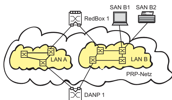
Abb. 35: Netz mit implementiertem Parallelredundanz-Protokoll
