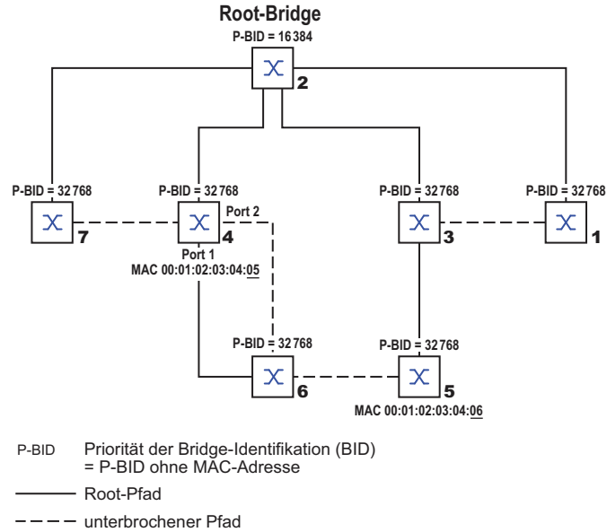
Abb. 48: Beispiel für die Manipulation der Baumstruktur
