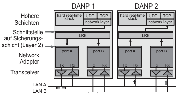
Abb. 34: Ablauf PRP/LRE
