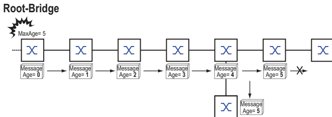
Abb. 44: Übertragung einer STP-BPDU in Abhängigkeit von MaxAge
