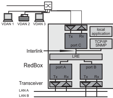
Abb. 36: RedBox-Umwandlung doppeltes auf einfaches LAN
