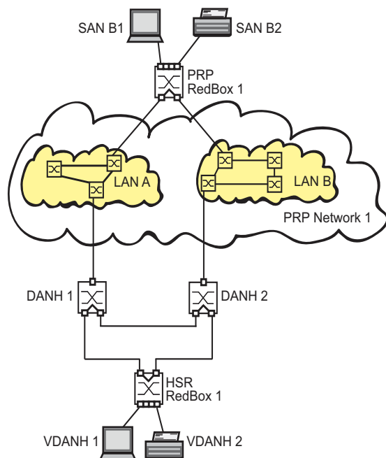
Abb. 39: PRP-Netz mit einem HSR-Netz verbinden
