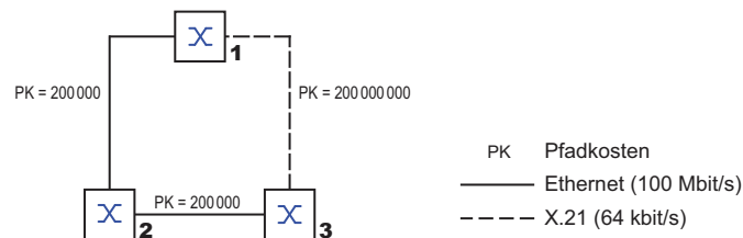
Abb. 41: Pfadkosten
