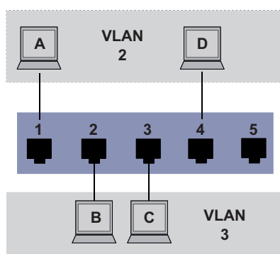
Abb. 26: Beispiel für ein einfaches Port-basiertes VLAN
