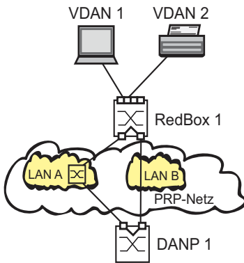
Abb. 37: Beispiel für ein PRP-Netz
