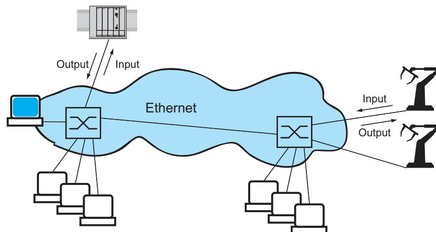
Abb. 47: Beispiel für die Kommunikation.
