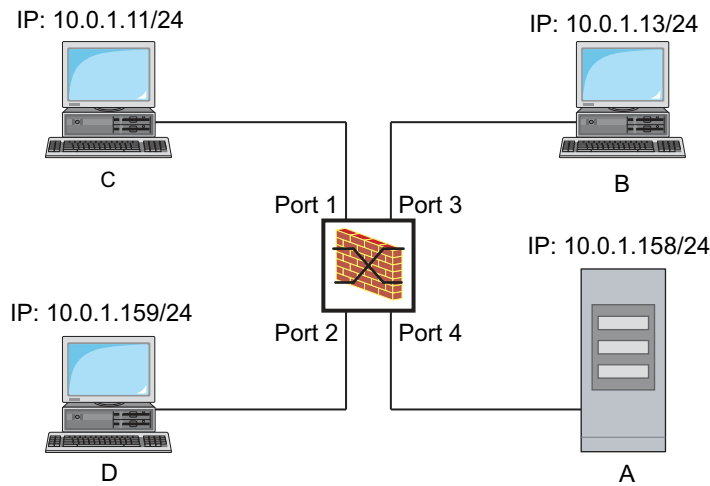
Abb. 19: Beispiel einer IP-ACL
