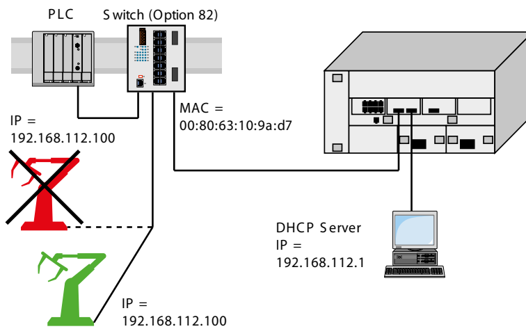
Abb. 65: Anwendungsbeispiel für den Einsatz von Option 82
