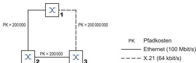
Abb. 32: Pfadkosten
