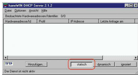
Abb. 56: Statische Adresseingabe
