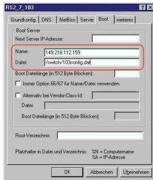
Abb. 54: Konfigurationsdatei auf dem tftp-Server
