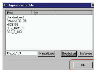
Abb. 55: Konfigurationsprofile verwalten
