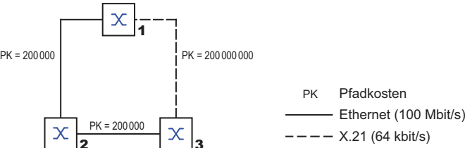
Abb. 37: Pfadkosten
