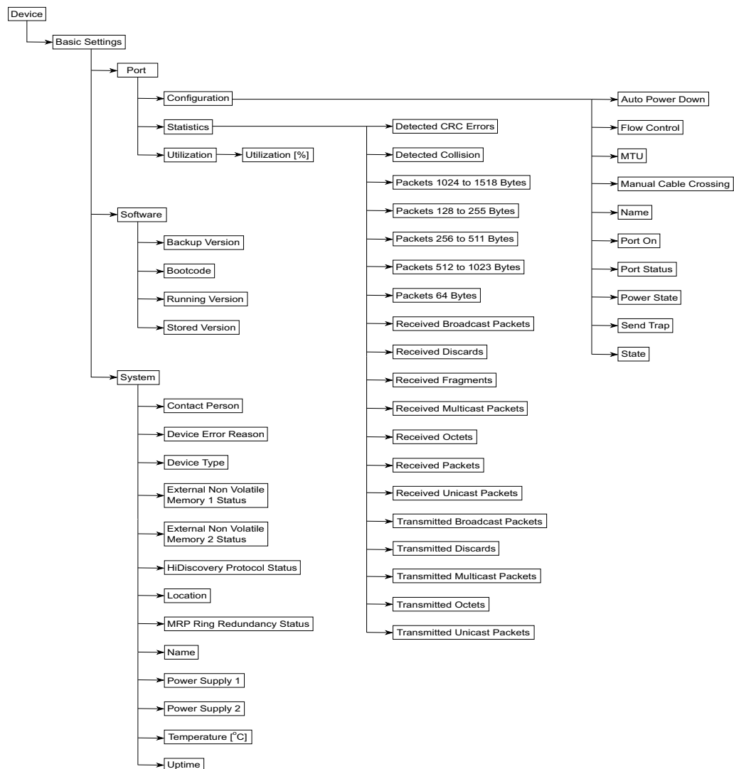
Abb. 79: OPC UA-Informationsmodell
