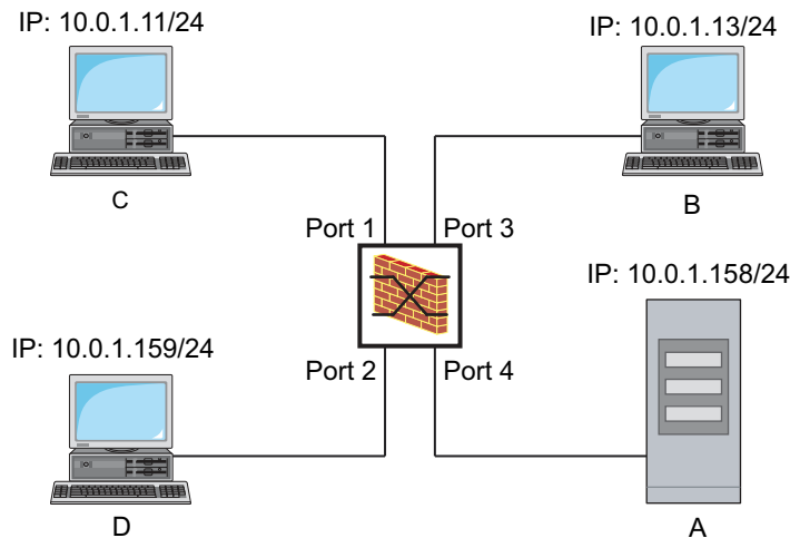
Abb. 20: Anwendungsbeispiel für eine IP-ACL
