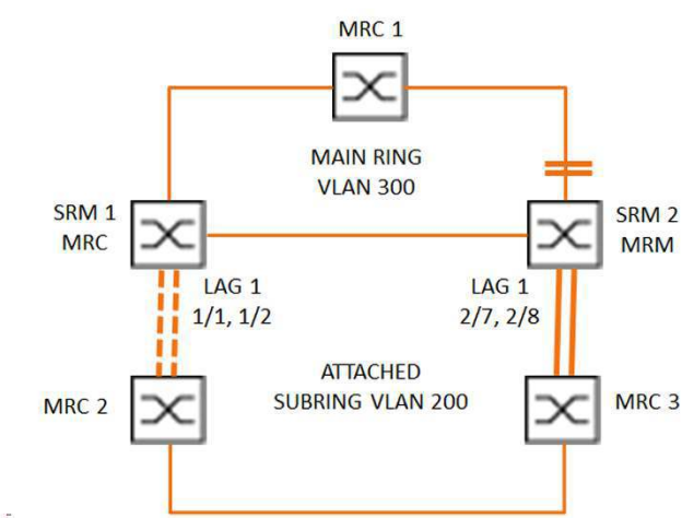
Abb. 54: Sub-Ring mit Link-Aggregation
