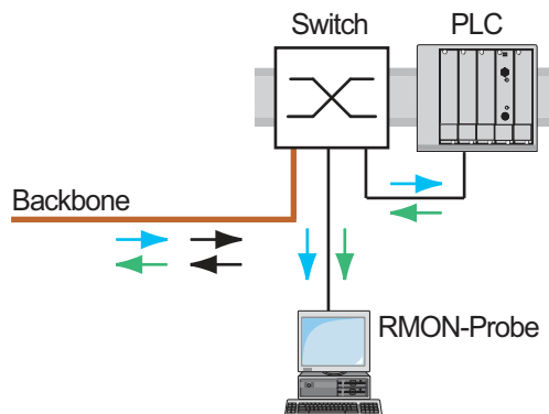
Abb. 72: Anwendungsbeispiel für ein Port-Mirroring-Setup
