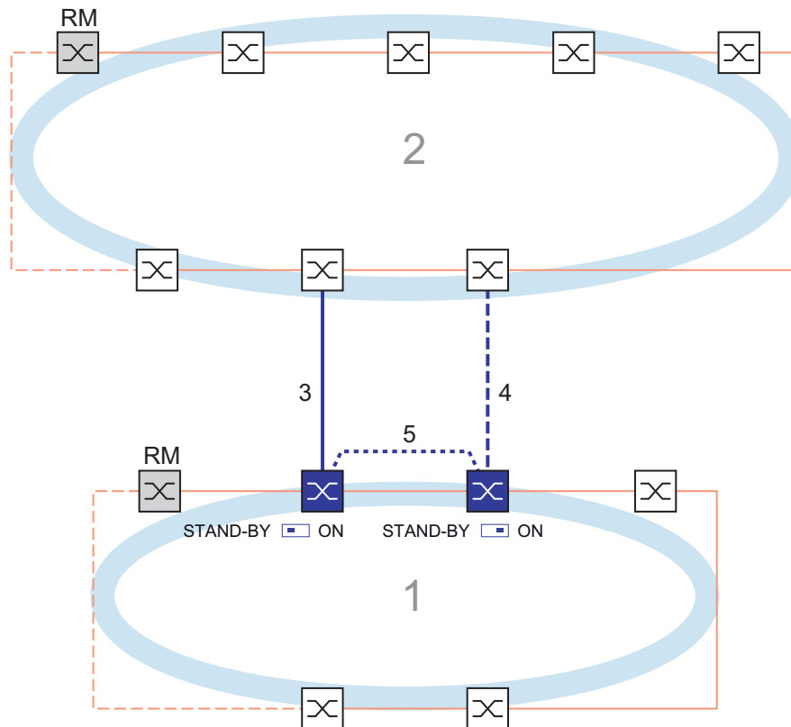
Abb. 67: Beispiel für die 2-Switch-Kopplung mit Steuerleitung
