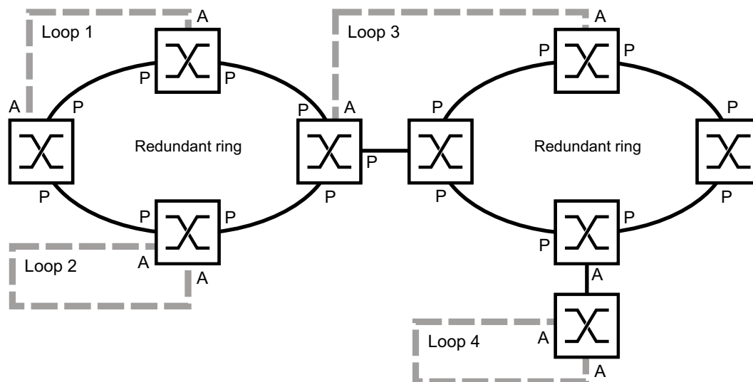
Abb. 71: Beispiele für unbeabsichtigte Schicht-2-Loops
