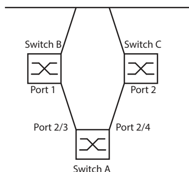
Abb. 47: Link-Backup Beispiel-Netzwerk
