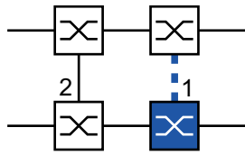
Abb. 58: 2-Switch-Kopplung, Standby-Gerät 1: Kopplungs-Port 2: Partner-Kopplungs-Port
