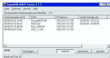
Abb. 90: DHCP-Server mit Einträgen
