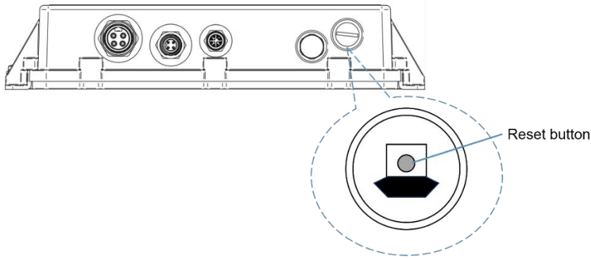
图 3: 复位按键
