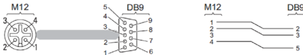
图 4: 用于连接外部管理站的终端电缆
