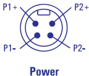
图 8: 电源插座的引脚分配
