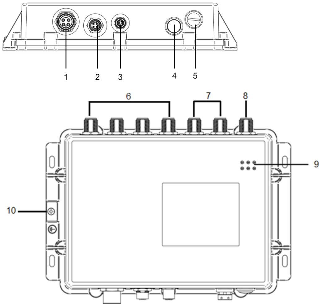
图 1: 设备视图
