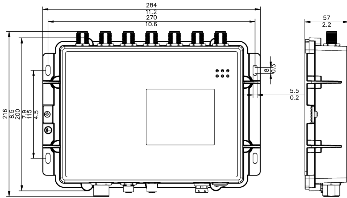
图 23: DAP847尺寸测量 (单位: \frac{mm}{inch} )
