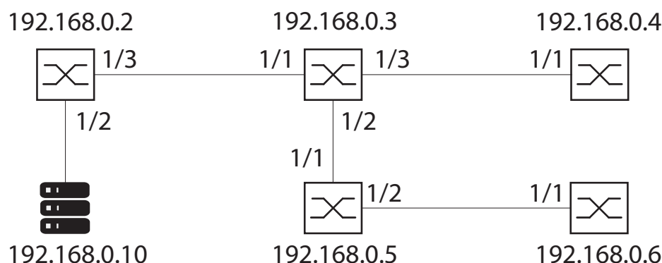
Figure 46 : Réseau avec serveur TFTP
