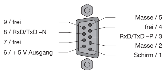
Abb. 2: Elektrischer Kanal– Anschlussbelegung Sub-D-Buchse (Bezeichnung entsprechend PROFIBUS-Norm)
